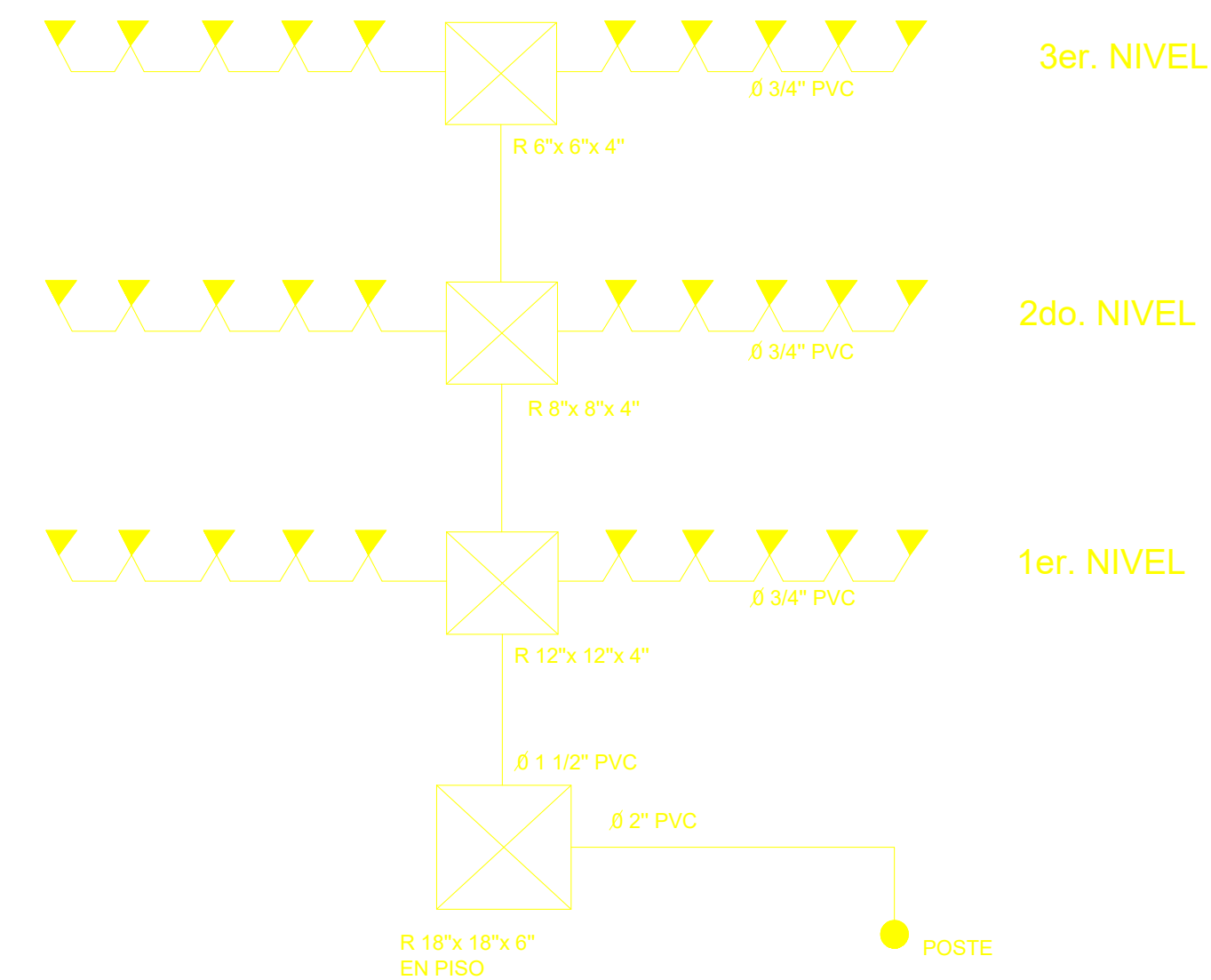
DIAGRAMA VERTICAL DE TELEFONO BLOQUE B
