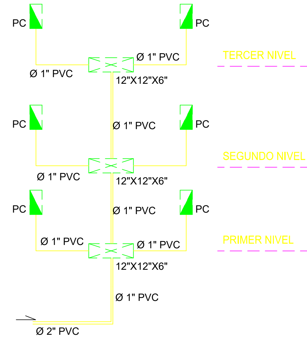
DIAGRAMA VERTICAL ELECTRICO BLOQUE B no escala
