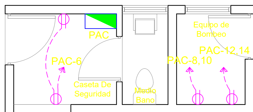
PLANTA TOMACORRIENTES CASETA GUARDIA Y EQUIPOS DE BOMBEO ESCALA: 1:40
