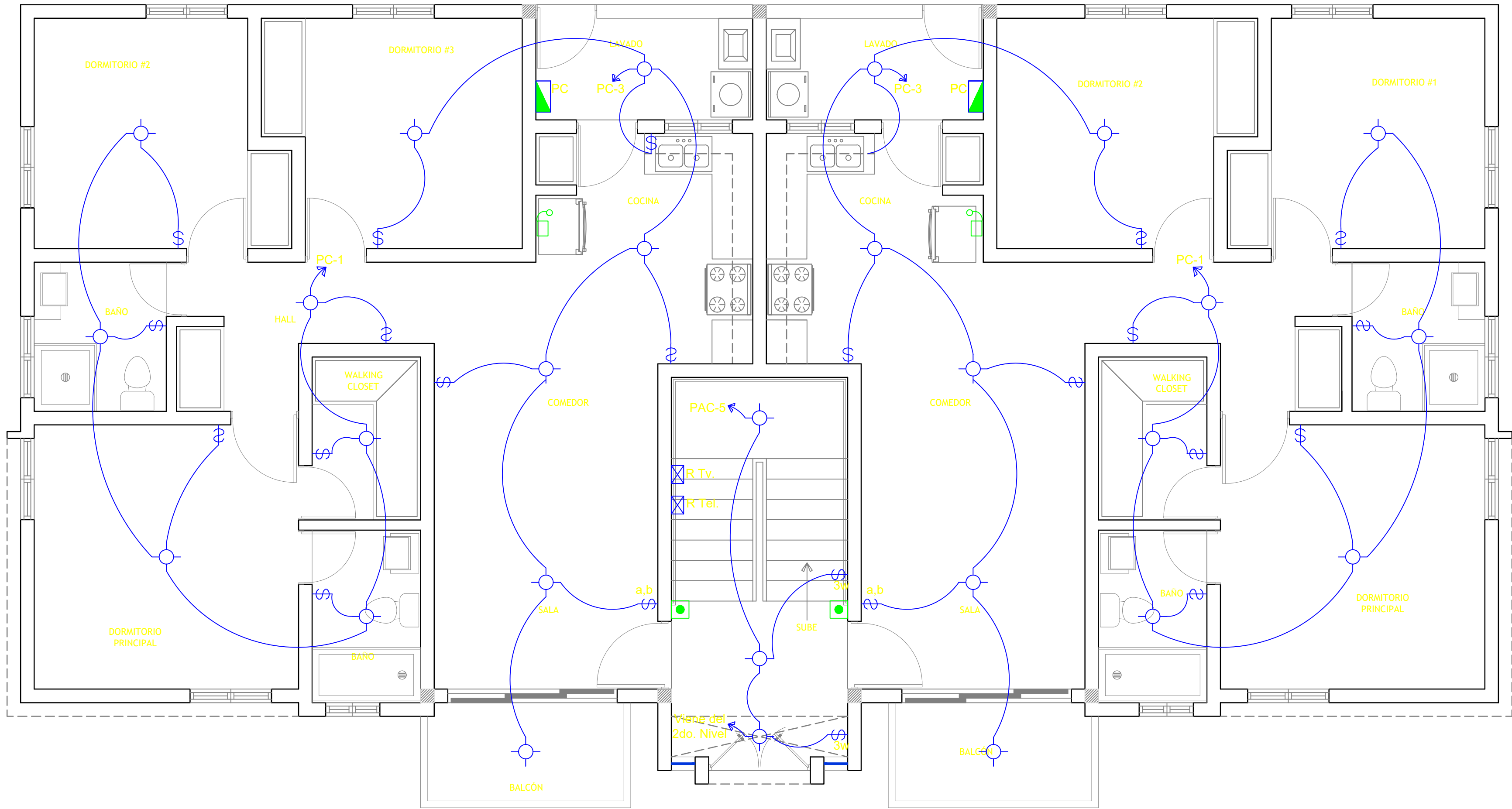
PLANTA LUMINARIAS 1ER. NIVEL, BLOQUE B ESCALA: 1:75
