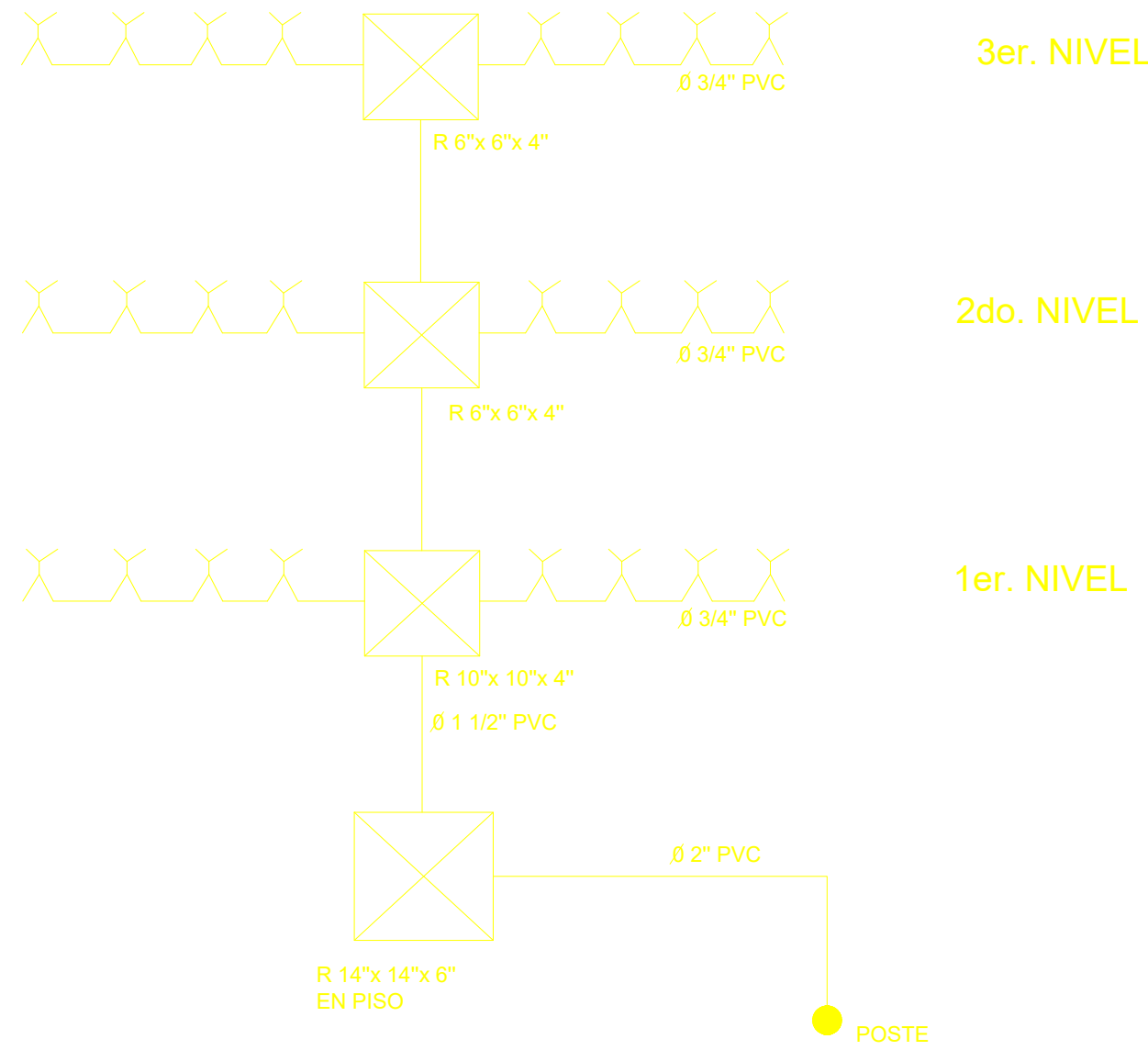
DIAGRAMA VERTICAL DE ANTENA BLOQUE B
