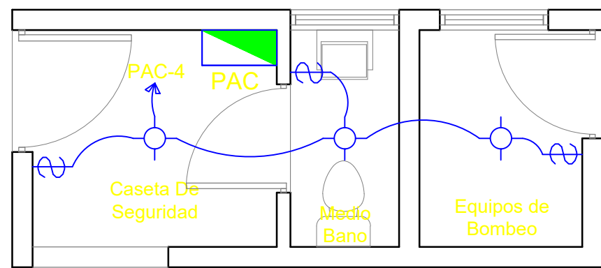
PLANTA LUMINARIAS CASETA GUARDIA Y EQUIPOS DE BOMBEO ESCALA: 1:40
